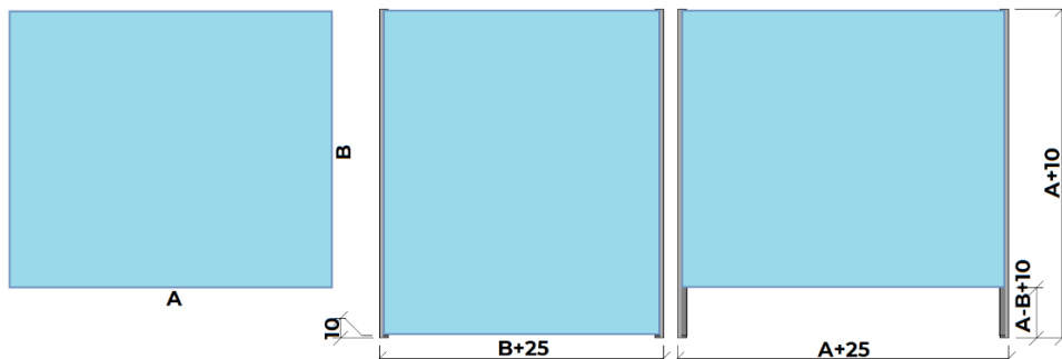
Montage PASSE-DOCUMENT
