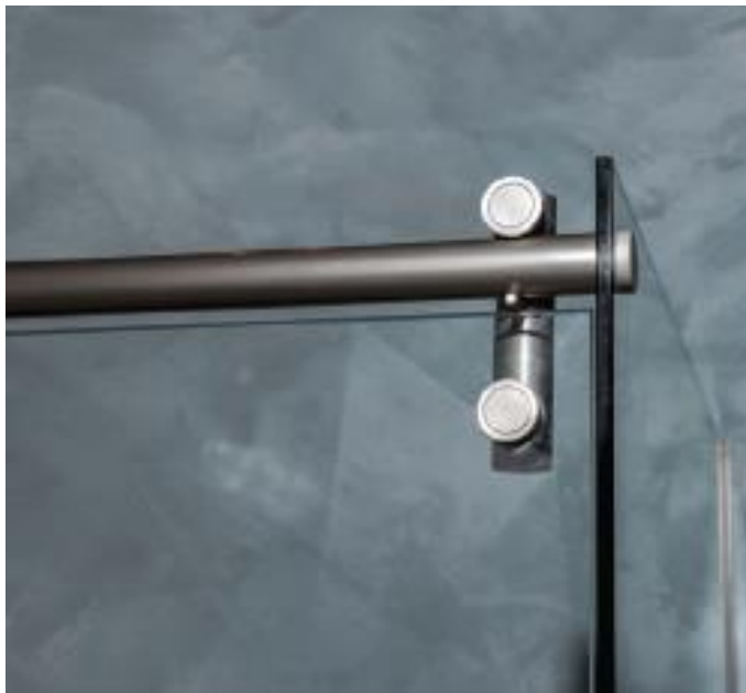
Detailansicht des Glas-Glas-Verbinders einer Eckkabine mit Gleitfront und fixem Seitenteil. Einfache Konzeption, klare Linien, effiziente Ausführung.
