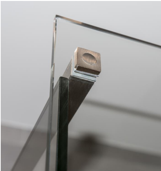
Quadratische Stabilisierungsstange Wand-Glas und Glas-Glas – Edelstahl gebürstet 20x20
