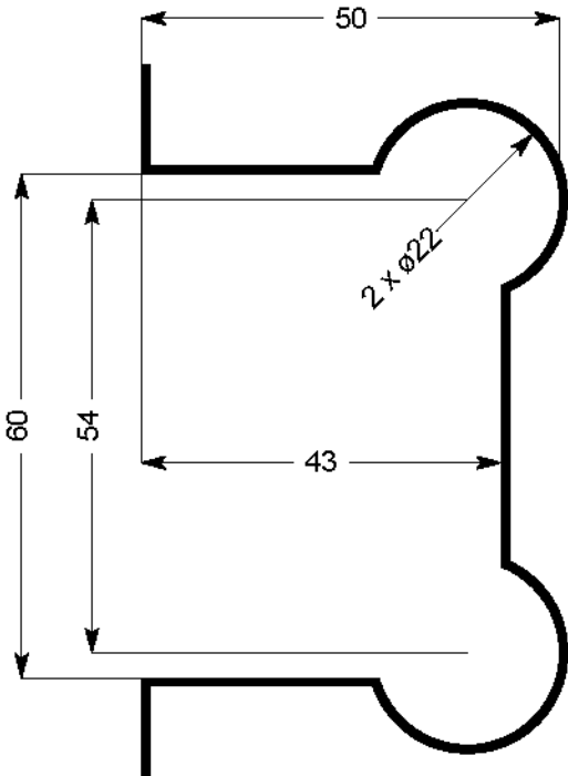
Encoche normale , écartement du support 6 mm Normal cutouts : 6 mm space between panels Encaje normal : distancia del soporte 6 mm Normaler Einschnitt : 6 mm Entfernung von Halter
