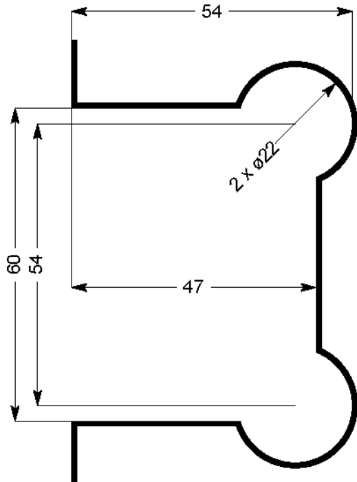
Encoche approfondie , écartement du support 2 mm Deeper cutout 2 mm space between panels Encaje profund distancia del soporte 2 mm Vertiefter Einschnitt : 2 mm Entfernung von Halter
